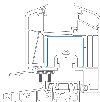
Hliníkový práh: výška 20 mm Obr.: 1:2
