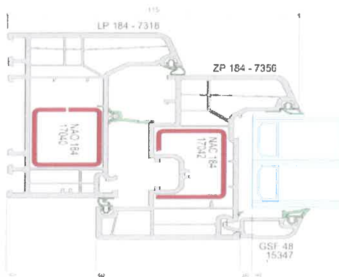
Obr. č. 1: výkres I (řez profilem)
